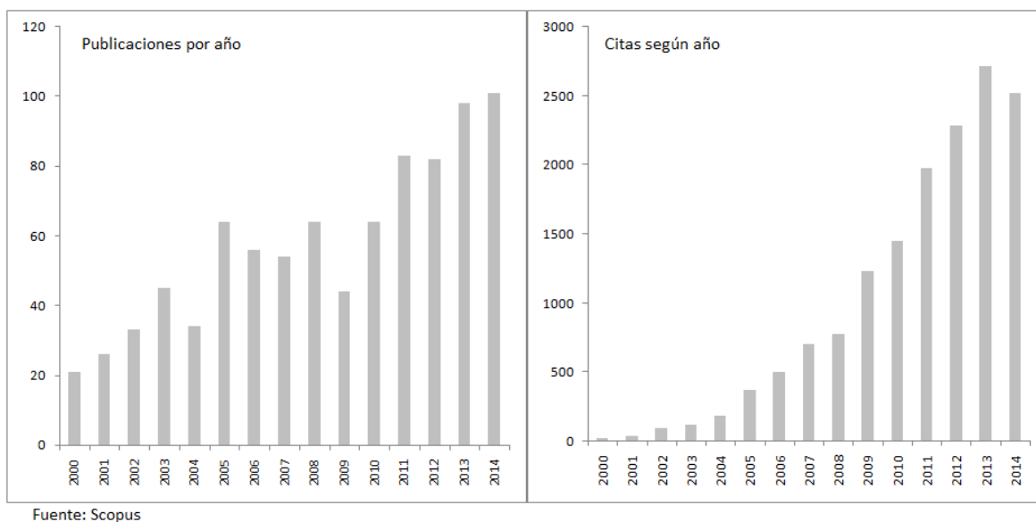
Figura 4.1.- Publicaciones y número de citas acumuladas por año de los miembros del Centro de Investigación Mente, Cerebro y Comportamiento desde 2000, según Scopus.
